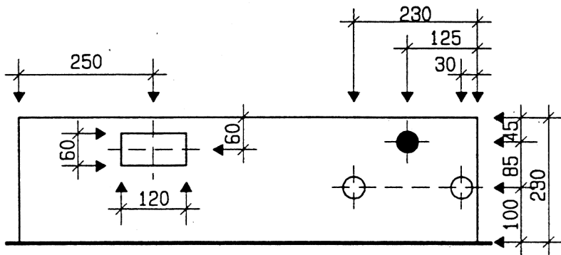
Ansicht oben
