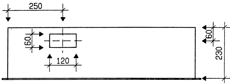
Ansicht oben
