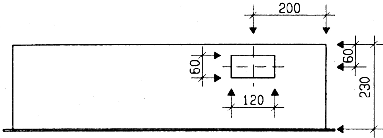
Ansicht oben
