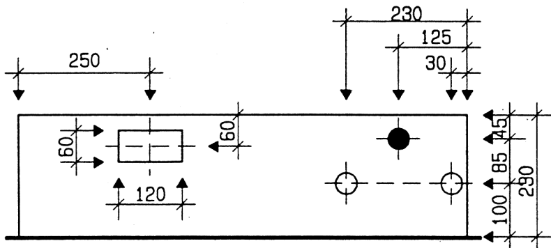
Ansicht oben
